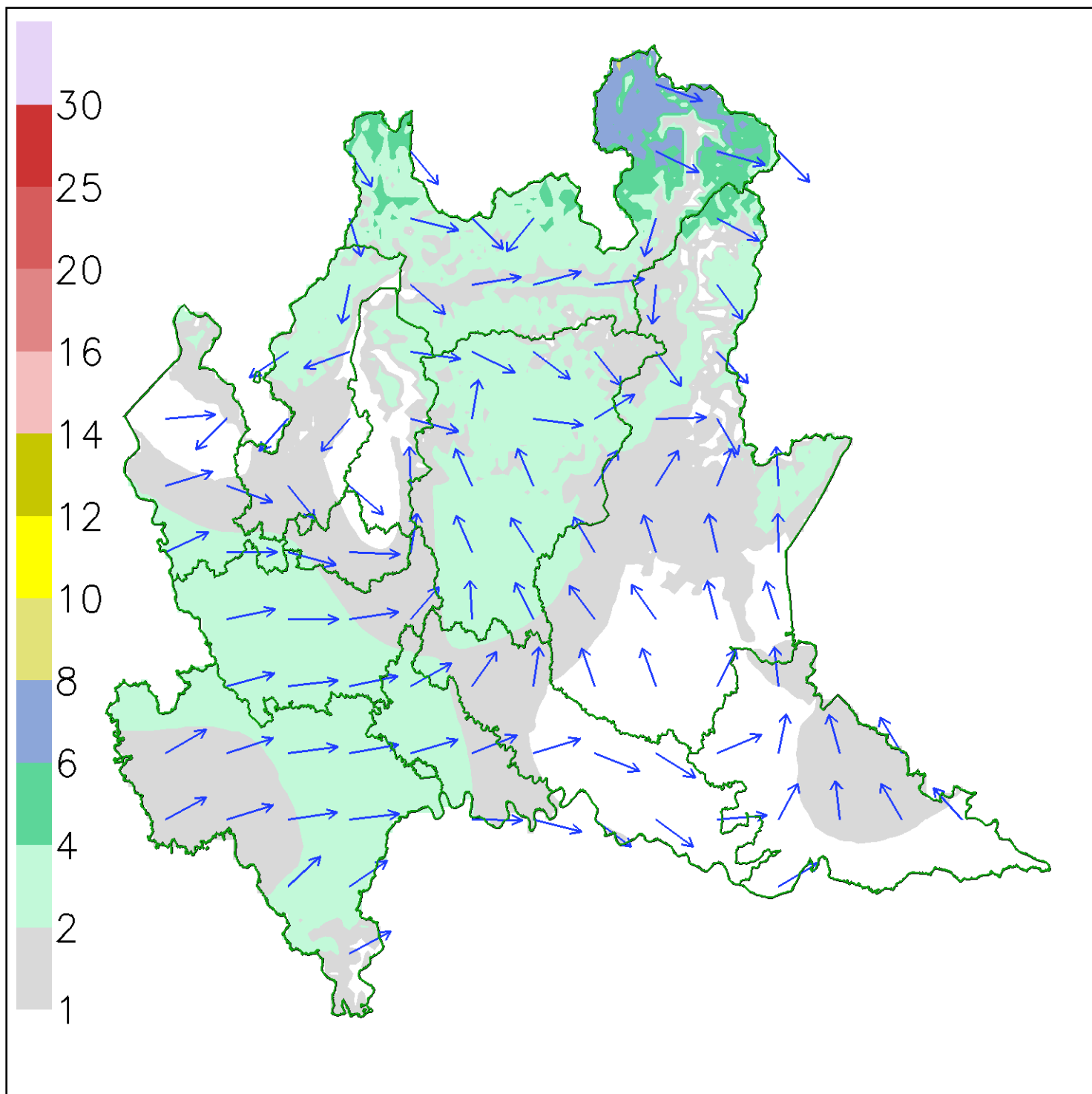
Vento medio orario m/s - ore 16
