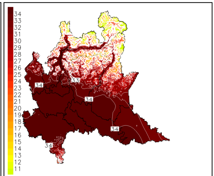
Temperature massime (°C)
