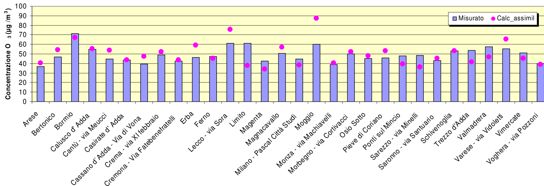
Figura A.3b: Concentrazione O 3 media annuale 2010 - Confronto misurato e calcolato senza assimilazione
