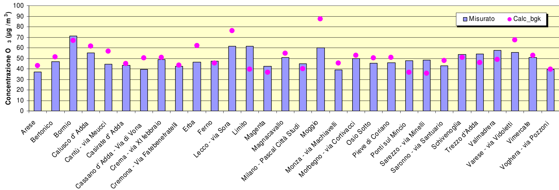
Figura A.3c: Concentrazione O 3 media annuale 2010 - Confronto misurato e calcolato background
