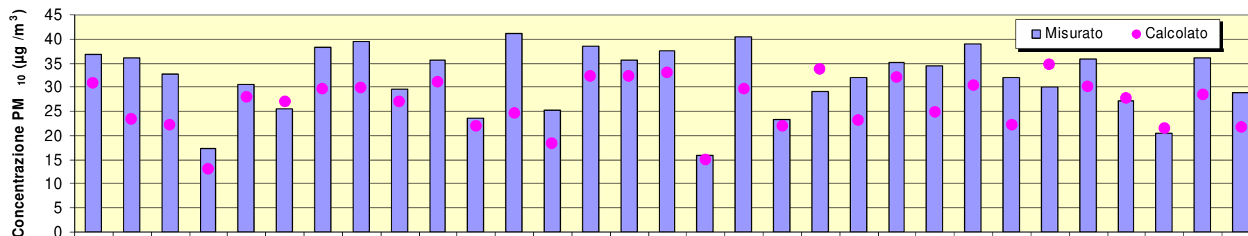
Figura A.1a: Concentrazione PM 10 media annuale 2010 - Confronto misurato e calcolato
