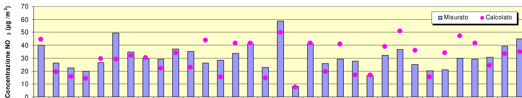
Figura A.2a: Concentrazione NO 2 media annuale 2010 - Confronto misurato e calcolato
