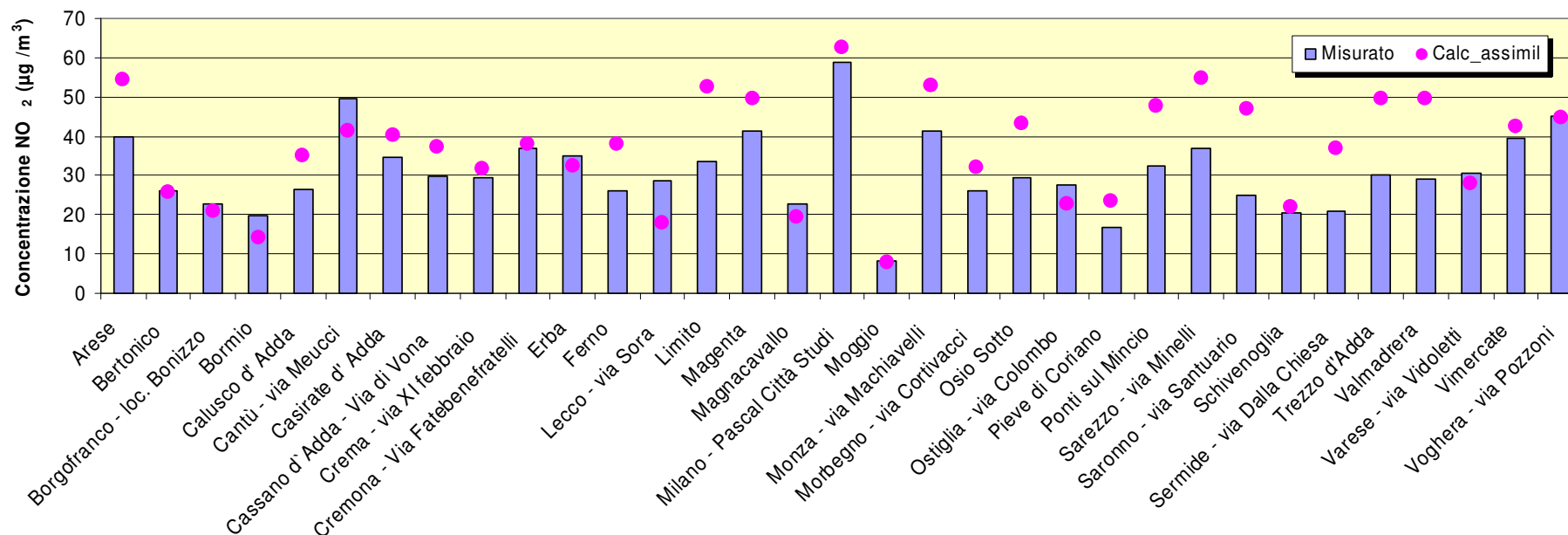
Figura A.2b: Concentrazione NO 2 media annuale 2010 - Confronto misurato e calcolato senza assimilazione
