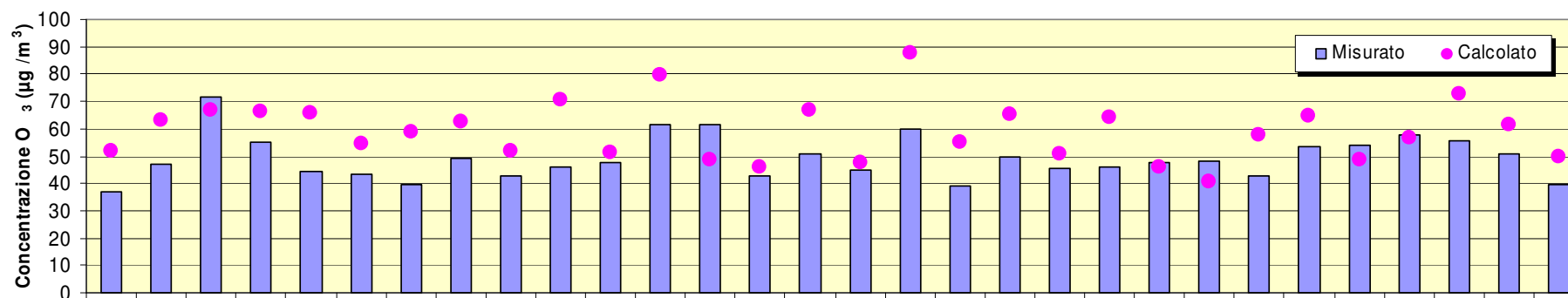
Figura A.3a: Concentrazione O 3 media annuale 2010 - Confronto misurato e calcolato
