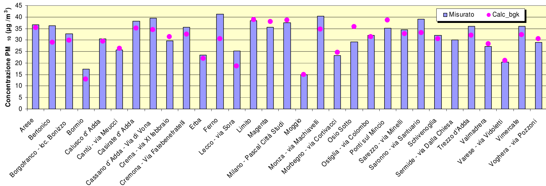
Figura A.1c: Concentrazione PM 10 media annuale 2010 - Confronto misurato e calcolato background
