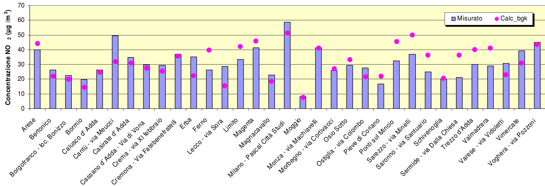
Figura A.2c: Concentrazione NO 2 media annuale 2010 - Confronto misurato e calcolato background
