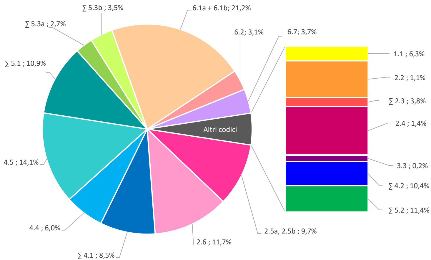
AI - FDM 2018
