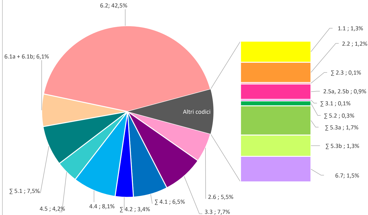
Tensioattivi - FDM 2018
