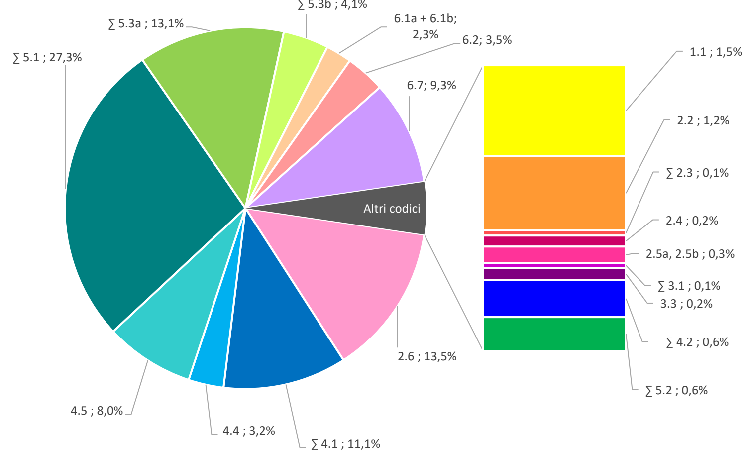
Ammoniaca - FDM 2018
