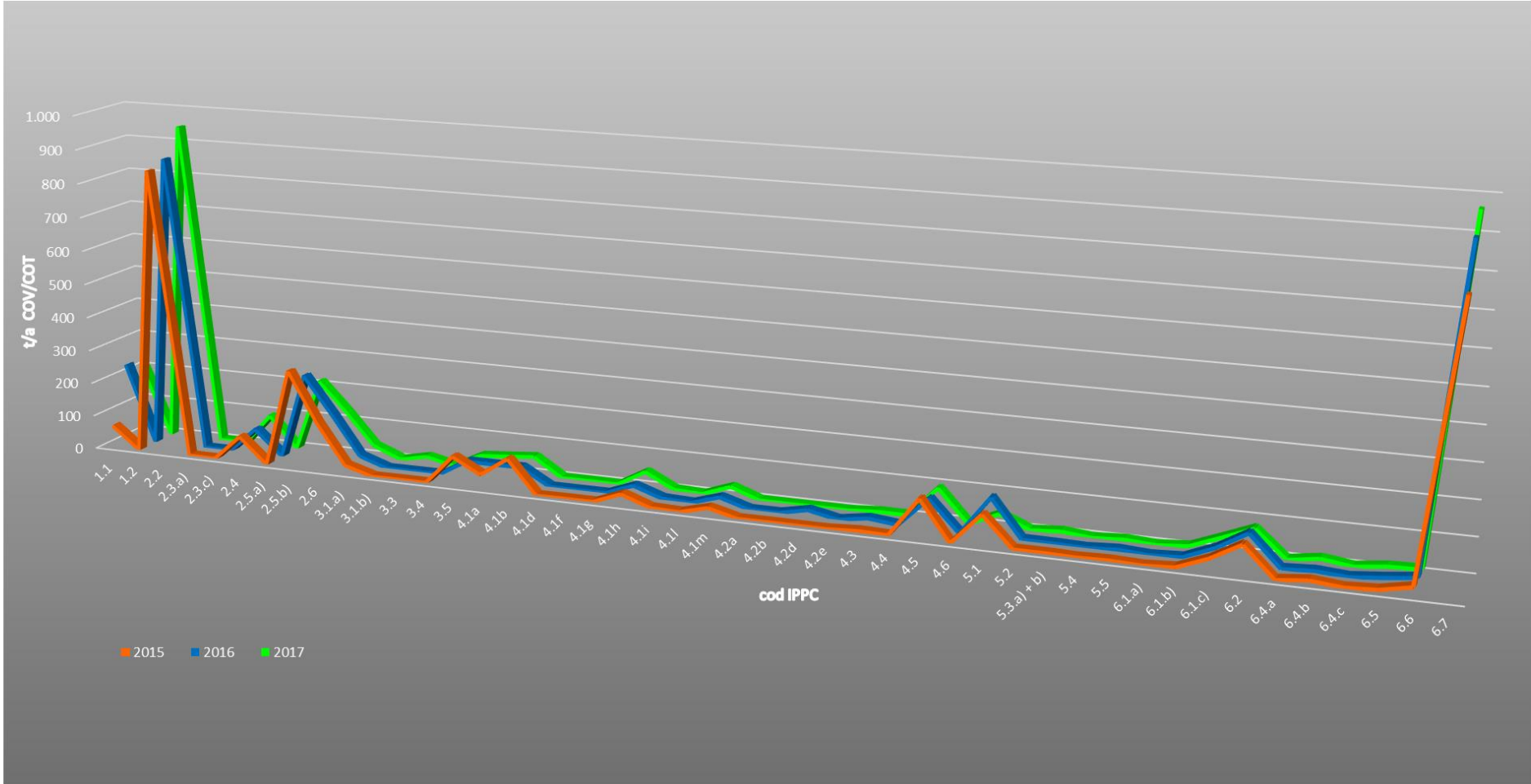
TREND EMISSIONI 2015/2017 - COV/COT
